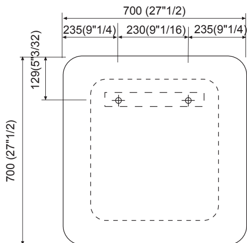
AMEM865Z
